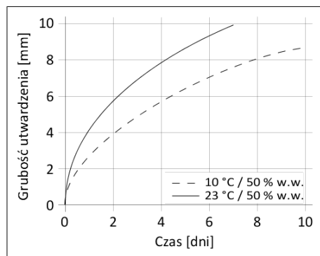
Diagram 1: Szybkość utwardzania Sikaflex®-221
